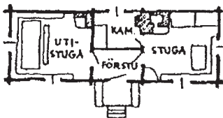
PARSTUGA
