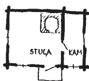
SIDOKAMMARSTUGA
